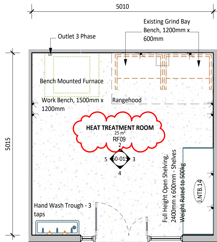
1 PLAN DETAIL 30-01 1 : 50
